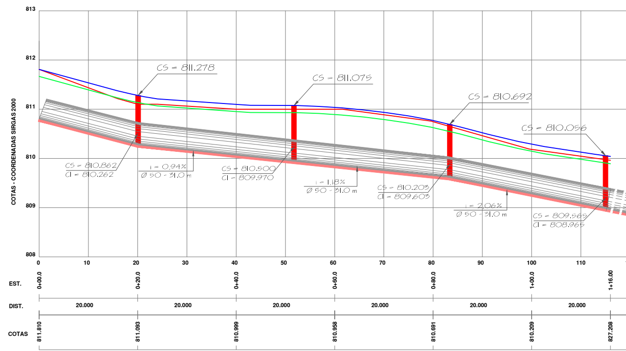
PERFIL LONGITUDINAL ESCALA HORIZONTAL 1:750 ESCALA VERTICAL 1:50
