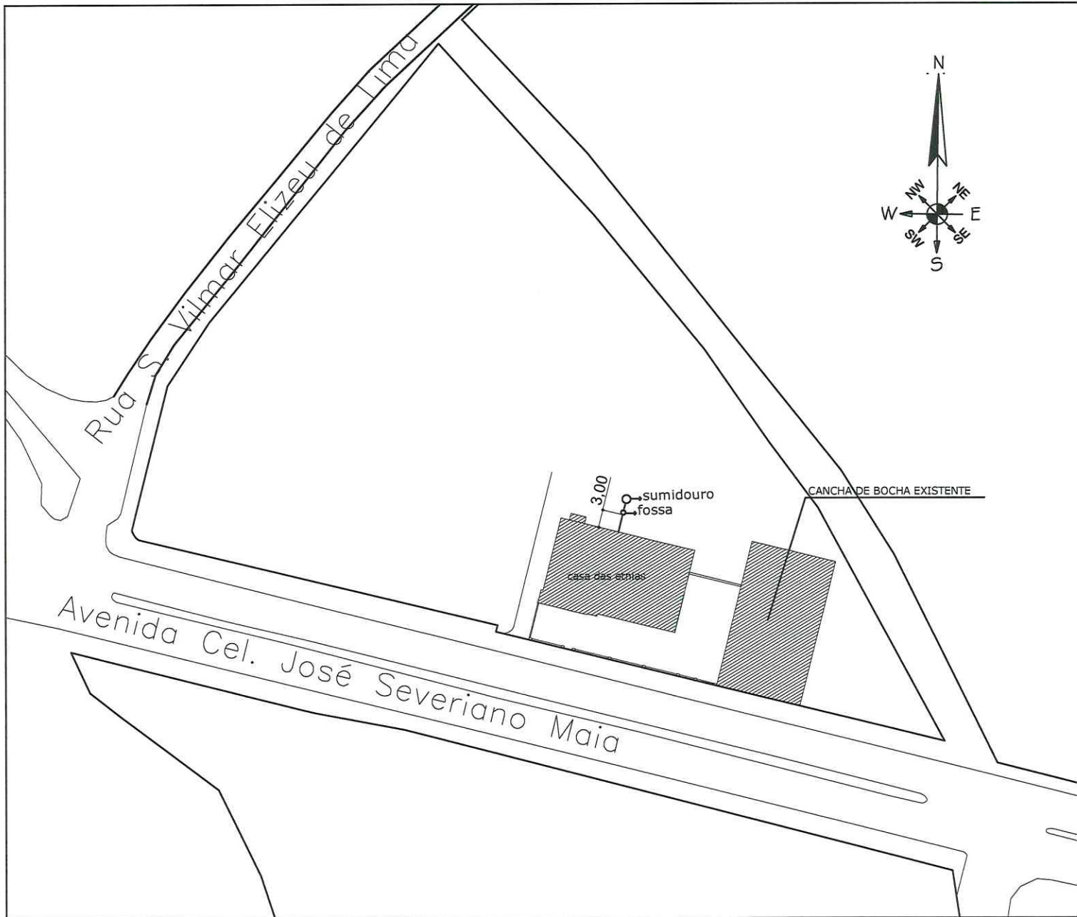
PLANTA DE SITUAÇÃO / ESCALA 1:1000
