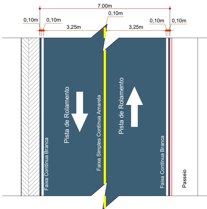
DETALHE DA SINALIZAÇÃO HORIZONTAL ESCALA: 1/100
