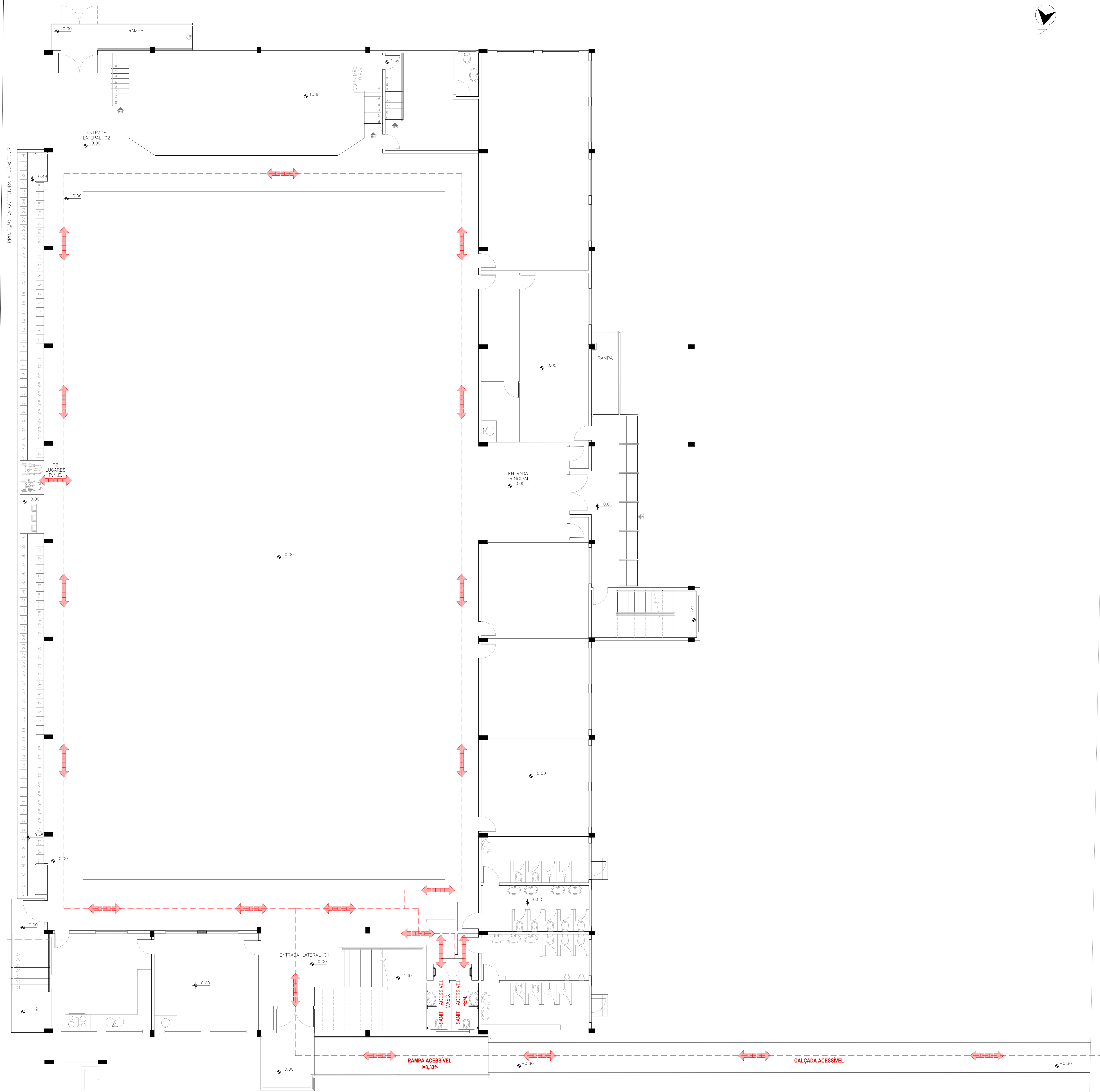
1 PLANTA DE ROTA ACESSÍVEL ESCALA 1:75
