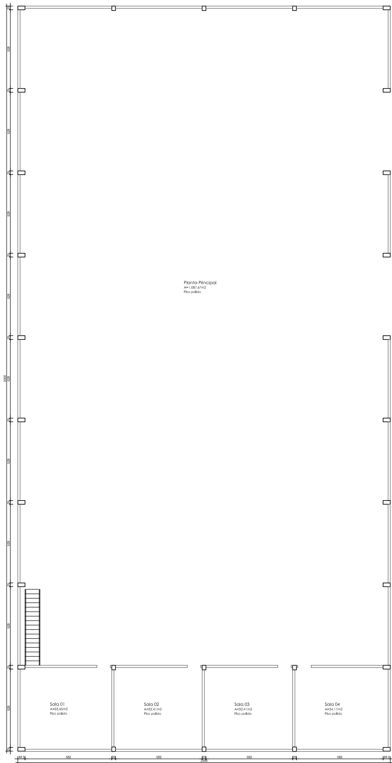
PLANTA BAIXA BARRACÃO Área total 1.250m² Escala 1:100
