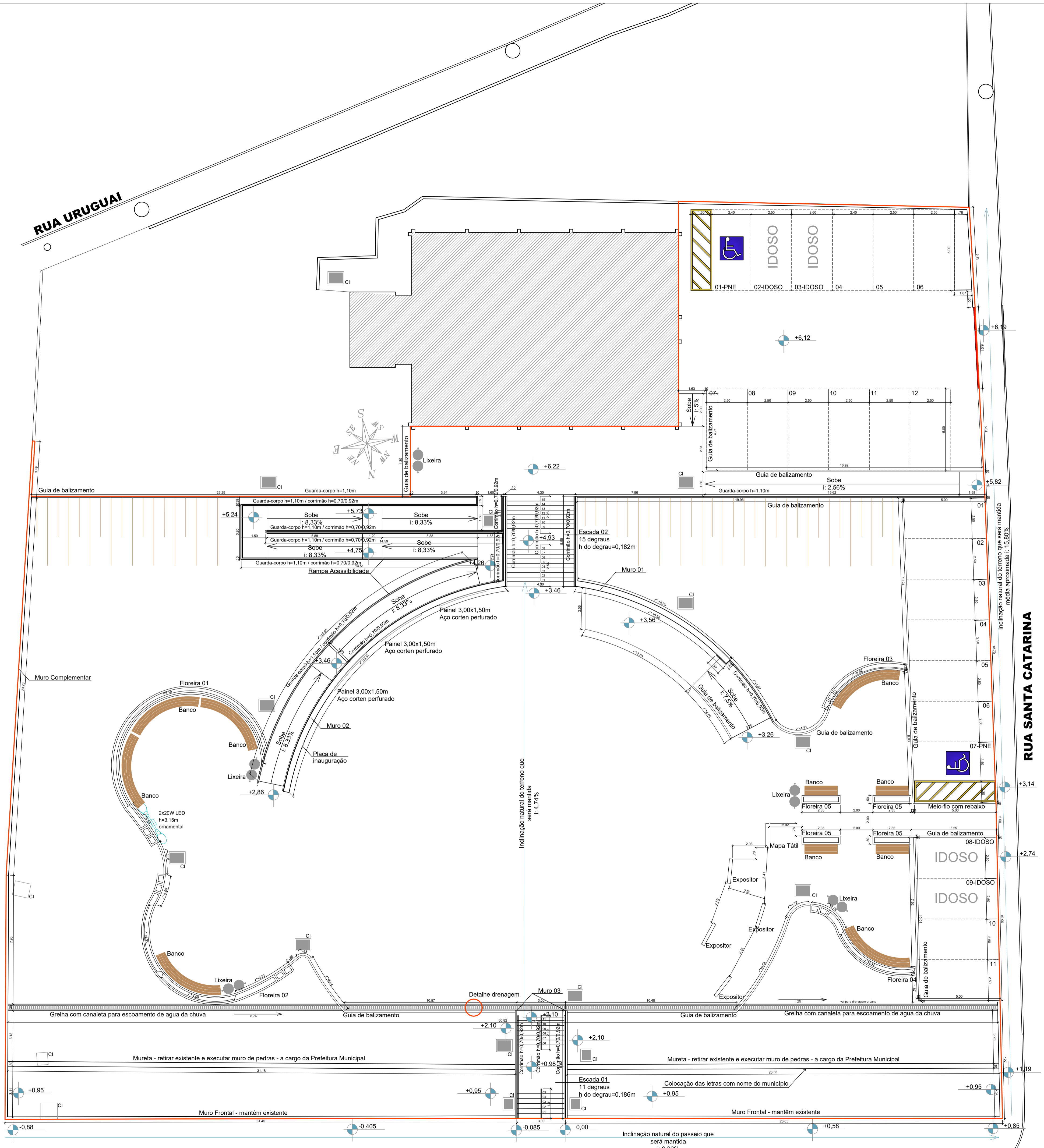
PLANTA TÉCNICA ESC 1/125
