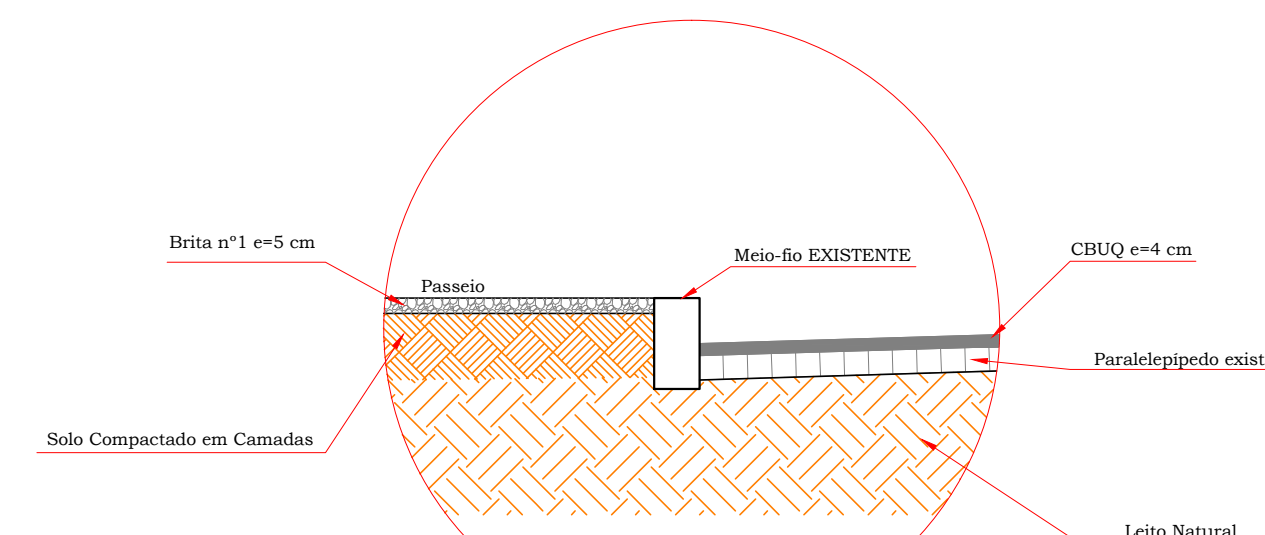
Detalhe 01 Escala 1:25
