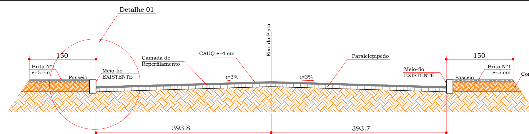
Seção Tipo (Seção 1: 2+11,79) Recapeamento Asfáltico Rua Governador Colombo Machado Salles Escala 1:50
