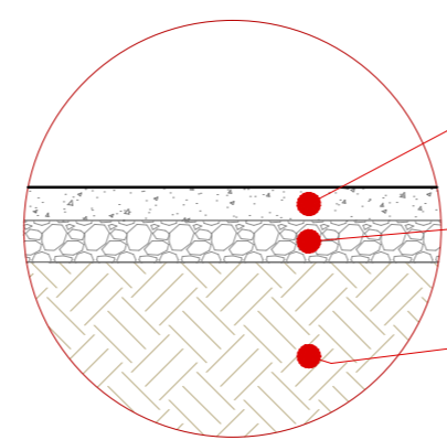
DETALHE 01 ESC:1/20
