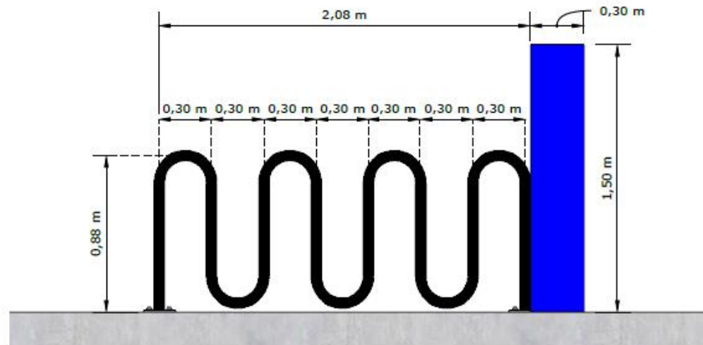
VISTA FRONTAL - MODELO 02 Escala: 1:20
