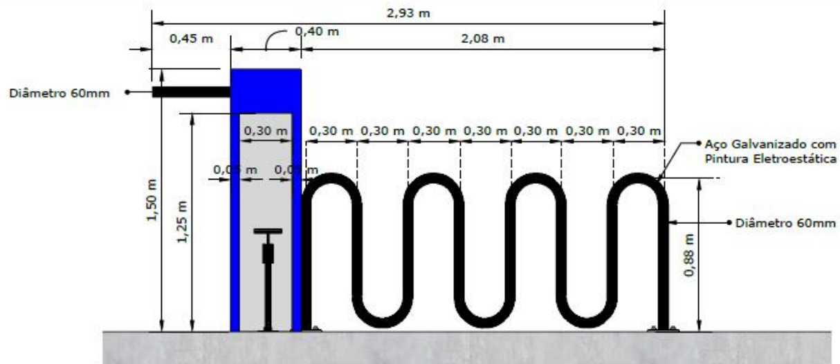
VISTA FRONTAL - MODELO 01 Esc.: 1:20
