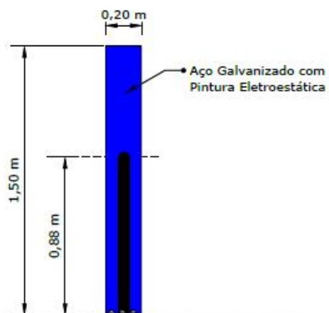
VISTA LATERAL DIREITA Escala: 1:20
