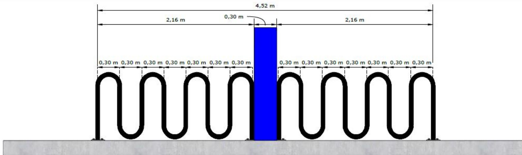
VISTA FRONTAL - MODELO 03 Esc.: 1:20
