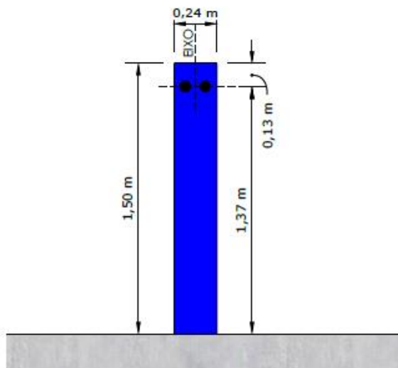
VISTA LATERAL ESQUERDA Esc.: 1:20
