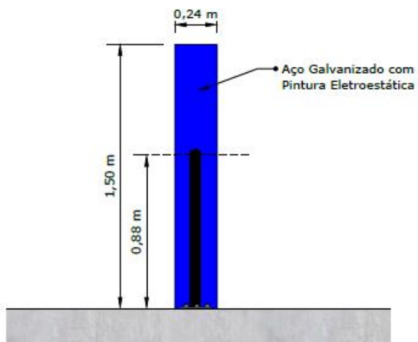
VISTA LATERAL DIREITA Esc.: 1:20
